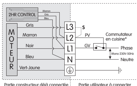
Schéma de câblage avec interrupteur
