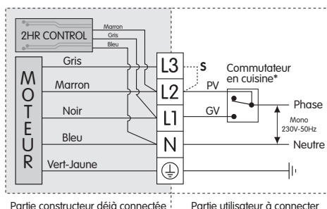
Schéma de câblage avec inverseur
