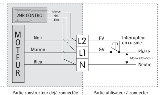
Schéma de câblage Bouton Poussoir
