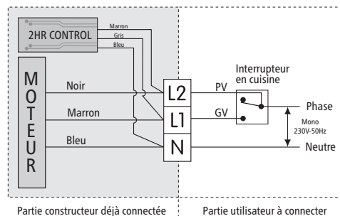
Schéma de câblage interrupteur va et vient
