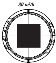
Partie à découper et retirer afin d'obtenir un piquage de 30m³/h. Utiliser un outil de découpe adapté et suivre le tracé carré.
