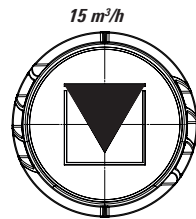
Partie à découper et retirer afin d'obtenir un piquage de 15m³/h. Utiliser un outil de découpe adapté et suivre le tracé triangulaire.
